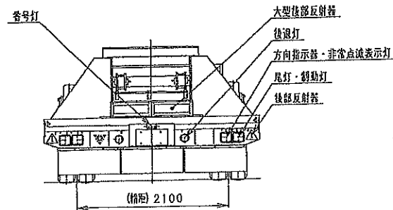
東邦TL47K0P3S型 セミトレーラ外觀四面図
